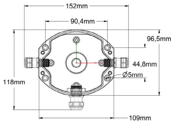
XT4* -BAL Boîtier IP65 aluminium
